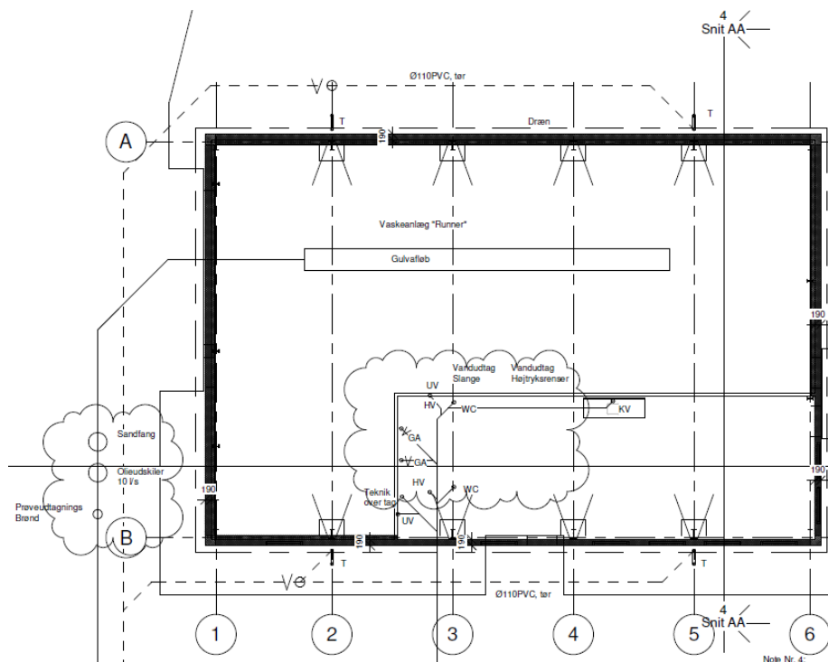
Afløbsplan for den ny Vaskehal med mandskabsfaciliteter på Delfinvej 12, 5800 Nyborg.
